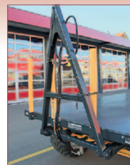
Klappbarer Deichsel mit verstellbarer Federentlastung.
